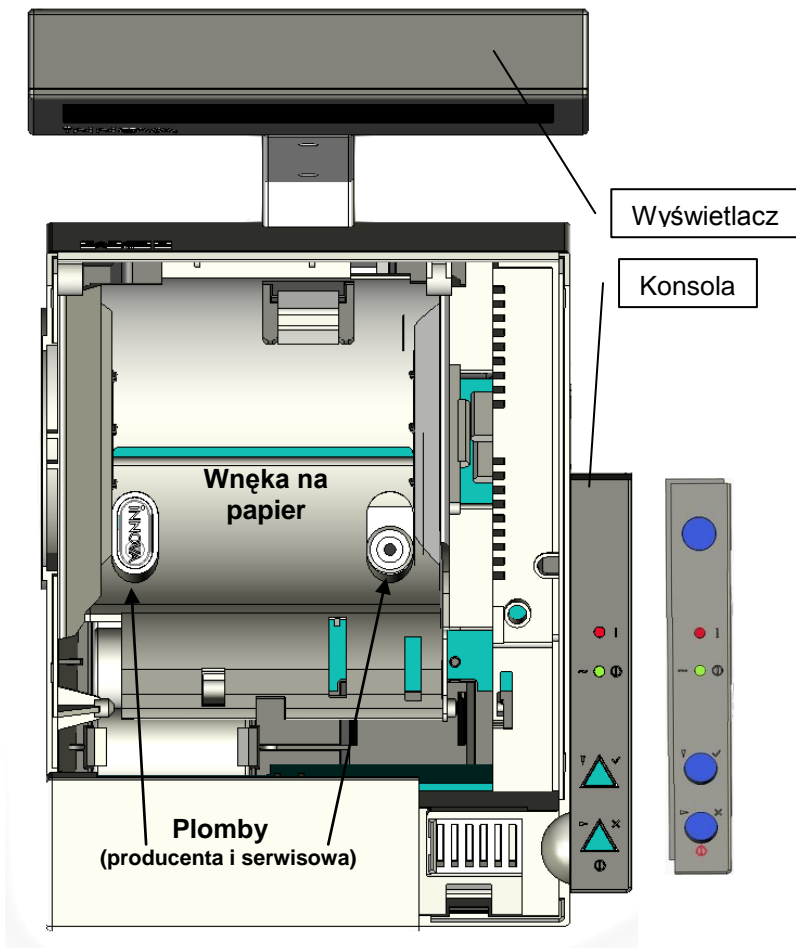
Rysunek 2. Budowa drukarki INNOVA DF-1
